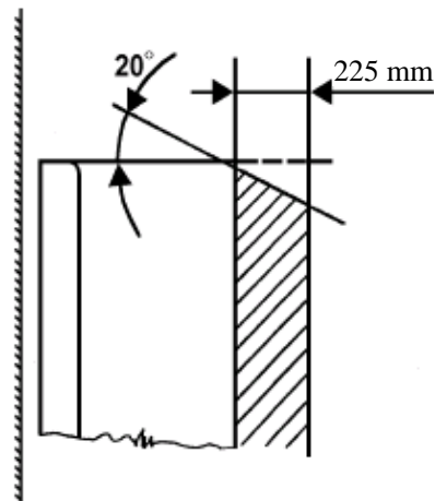
Longitudinal seat
